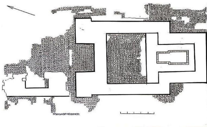
3 сызба - Қышқала қалашығынан анықталған №1 кесене. (Елеуов т.б. 2021: 91)
