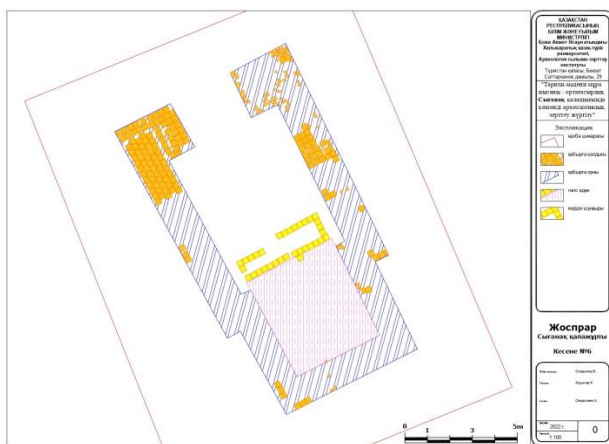
1 сызба - Сығанақ қалашығы №6 кесене.
